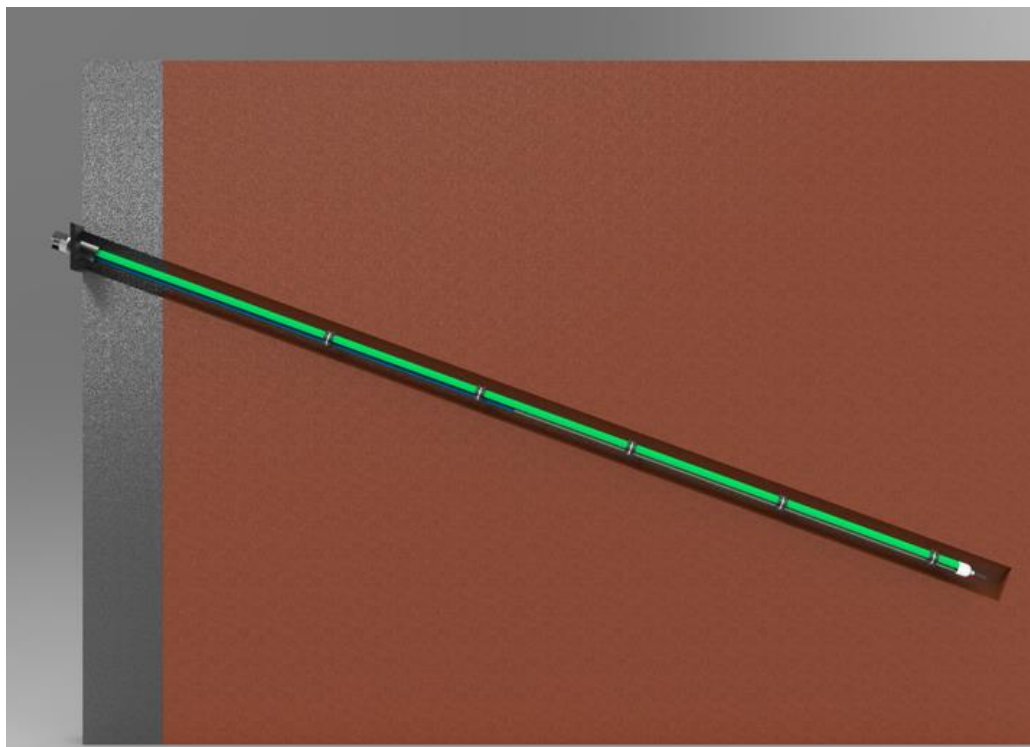
Anclaje Permanente - Inyección Global Única a 0 grados
