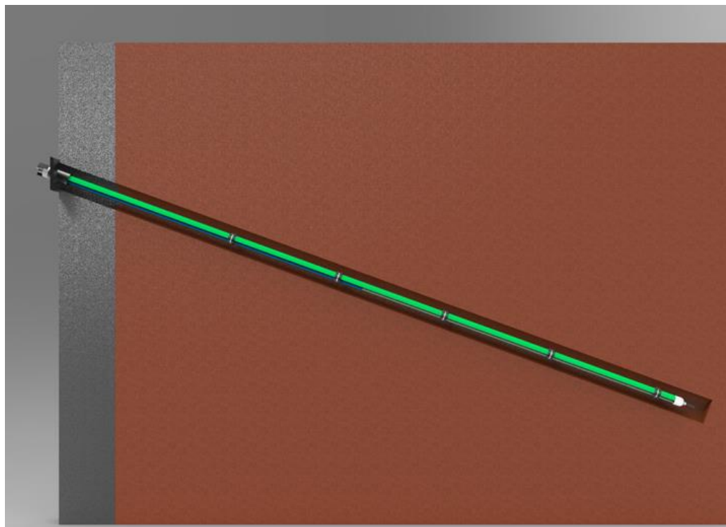
Ancoraggio permanente - Singola iniezione globale a 40 gradi
